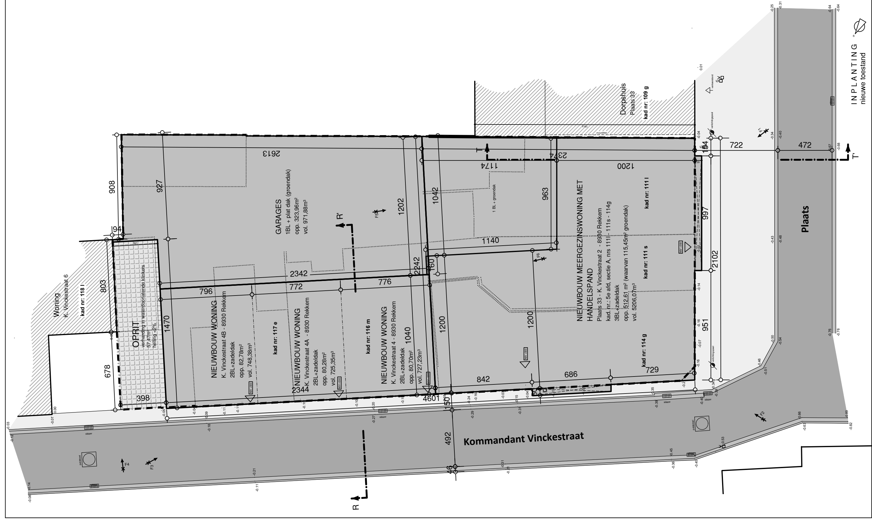
INPLANTING SCHAAL 1/200
